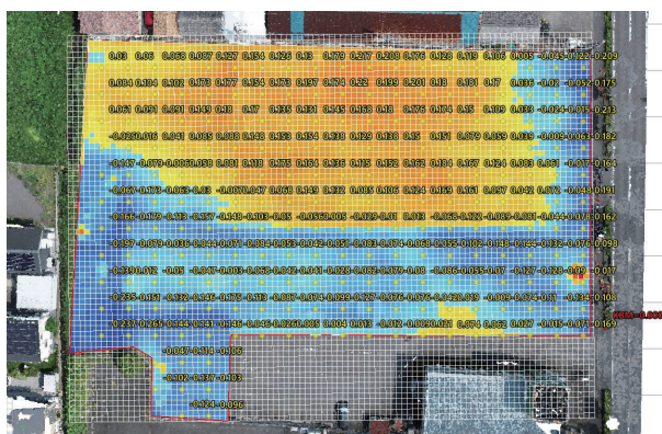
計測レベルを算出した点群データ
