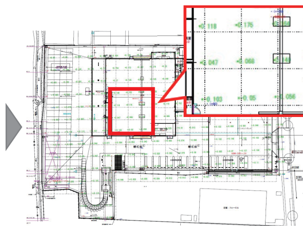
算出したレベルの数値を載せた図面
